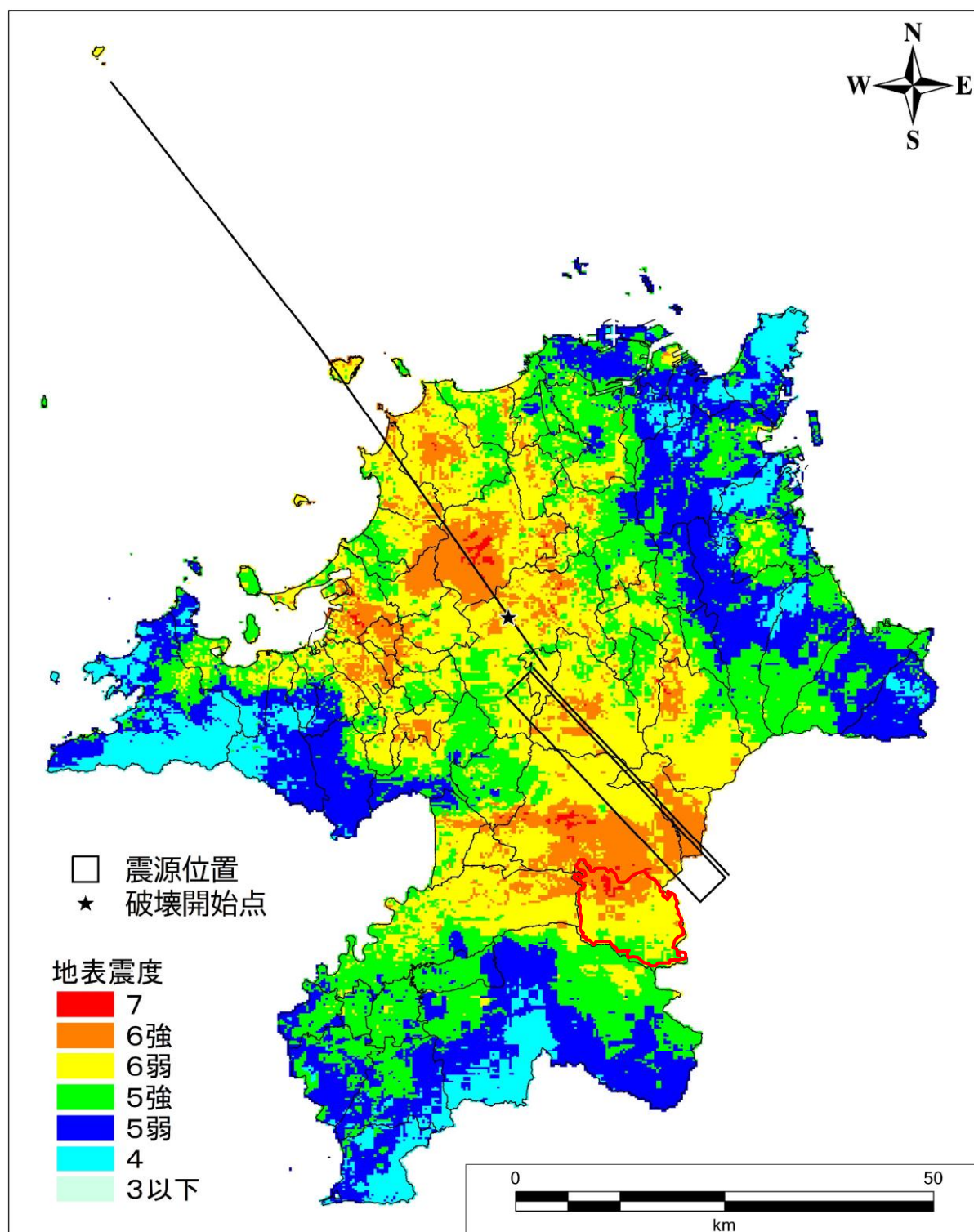
地表震度分布図【西山断層帯連動（大島沖区間＋西山区間＋嘉麻峠区間）（破壊開始点：中央）】
