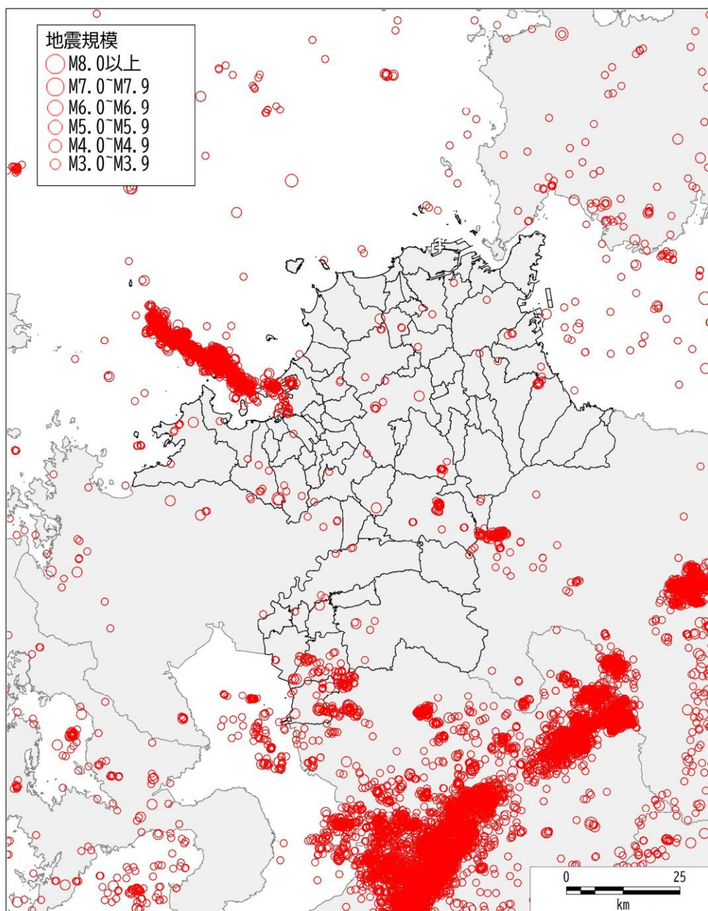
近年の福岡県周辺の震央分布図
