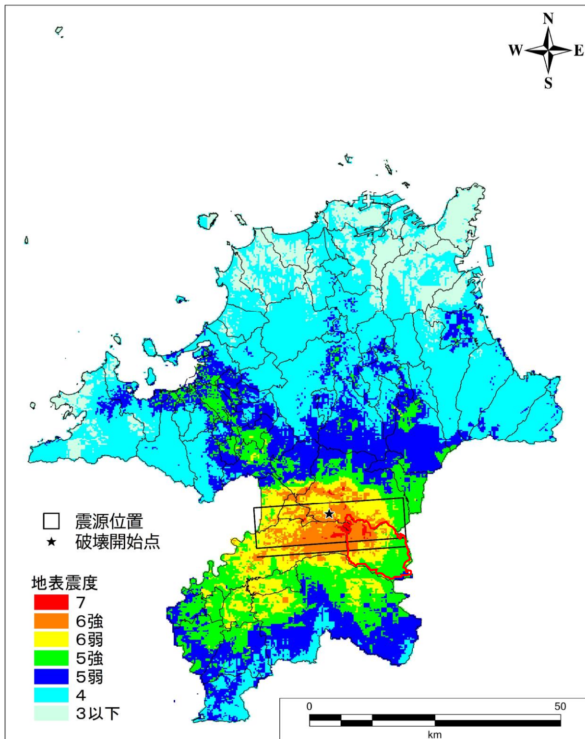
地表震度分布図【水縄断層帯（破壊開始：中央）】
